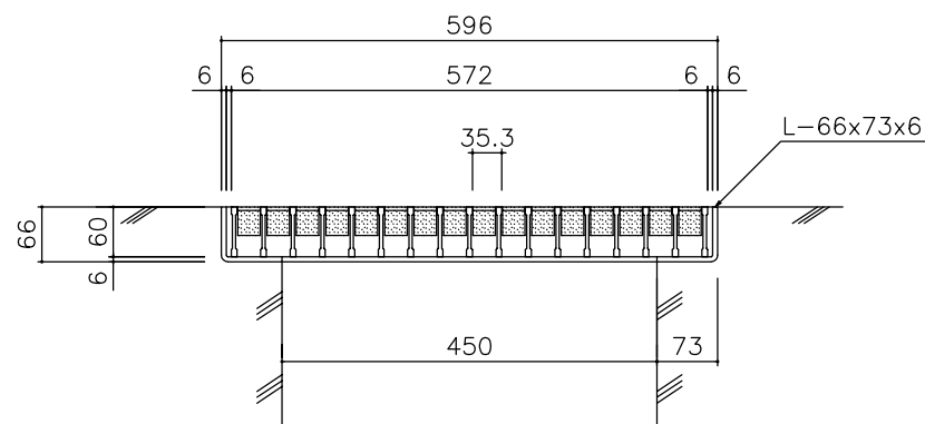
越流抑制グレーチング ヨドウォーターフォールズ
