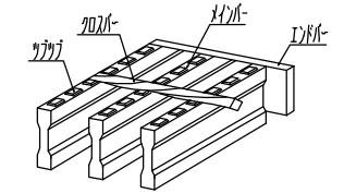
ツツブグレーチング
