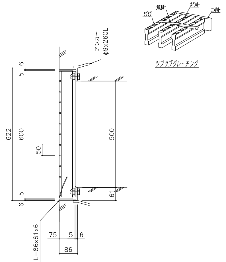
越流抑制グレーチング ヨドウォーターフォールズ
