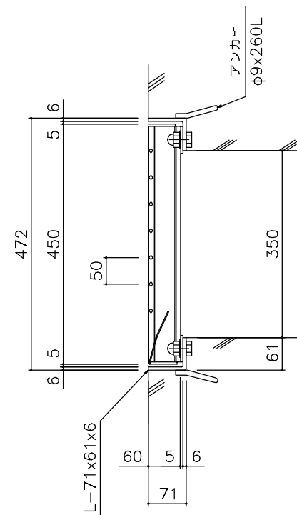
ツブツブグレーチング
