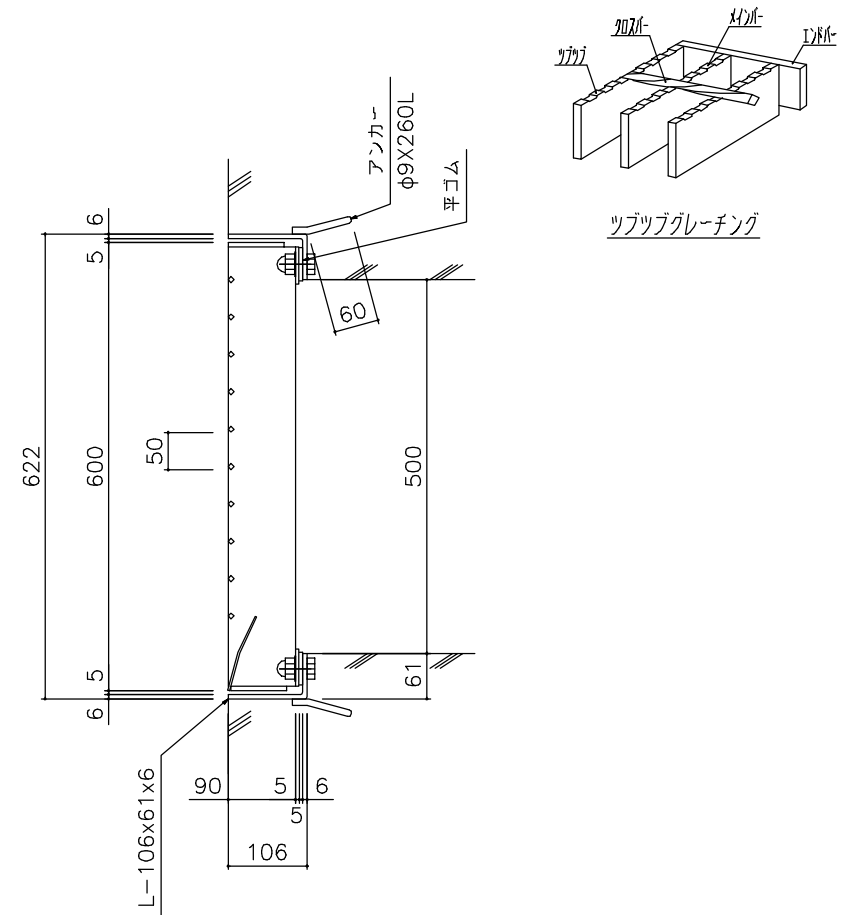
越流抑制グレーチング ヨドウォーターフォールズ
