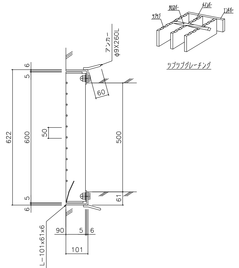
越流抑制グレーチング ヨドウォーターフォールズ
